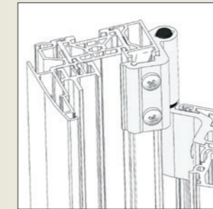
Paumelle à clamer
